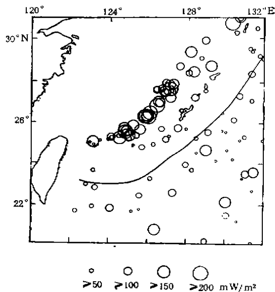
图5 热流分布
