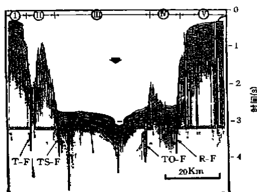
图3 横穿海槽南部的地震剖面 〔1〕
