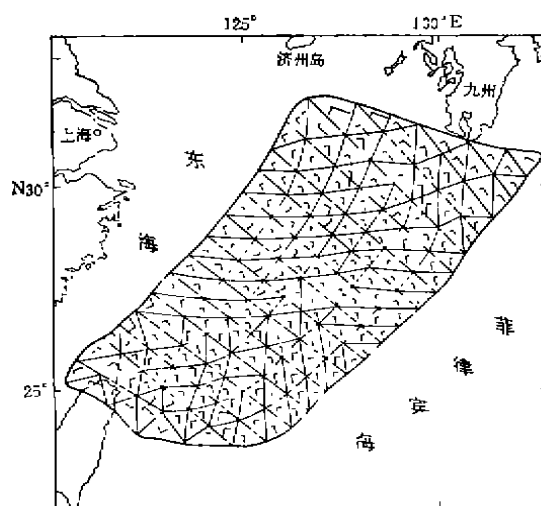
图2 上新世末主应力图(三角形网络为计算单元划分)
