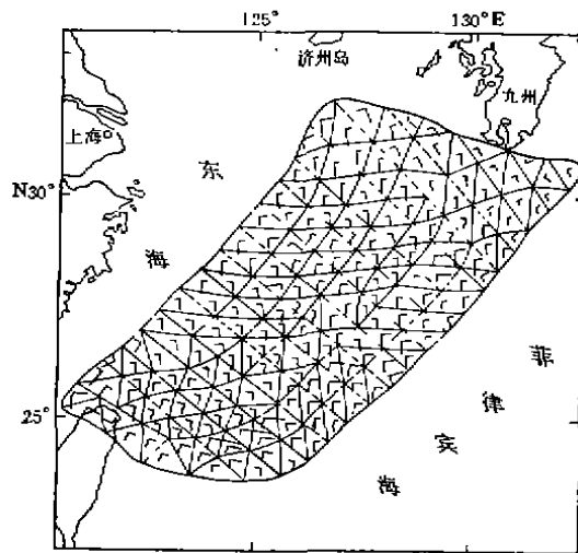
图 8 中新世末主应力(三角形网格为计算单元划分)
