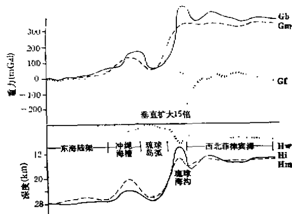
图 1 冲绳海槽地壳厚度剖面
