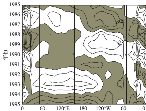
图5 1985—1995年有效波高(SWH)沿56°S纬圈的年距平(单位:m)分布特征(阴影部分代表负距平,50°~150°E对应的是印度洋的特征,150°E~60°W对应的是太平洋的特征,60°W~50°E对应的是大西洋的特征)
