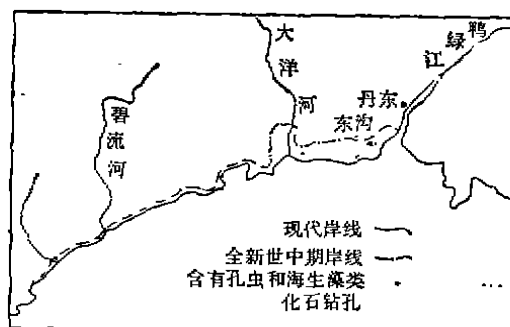
图 4 辽东半岛东部沿岸全新世中期海侵岸线位置图
