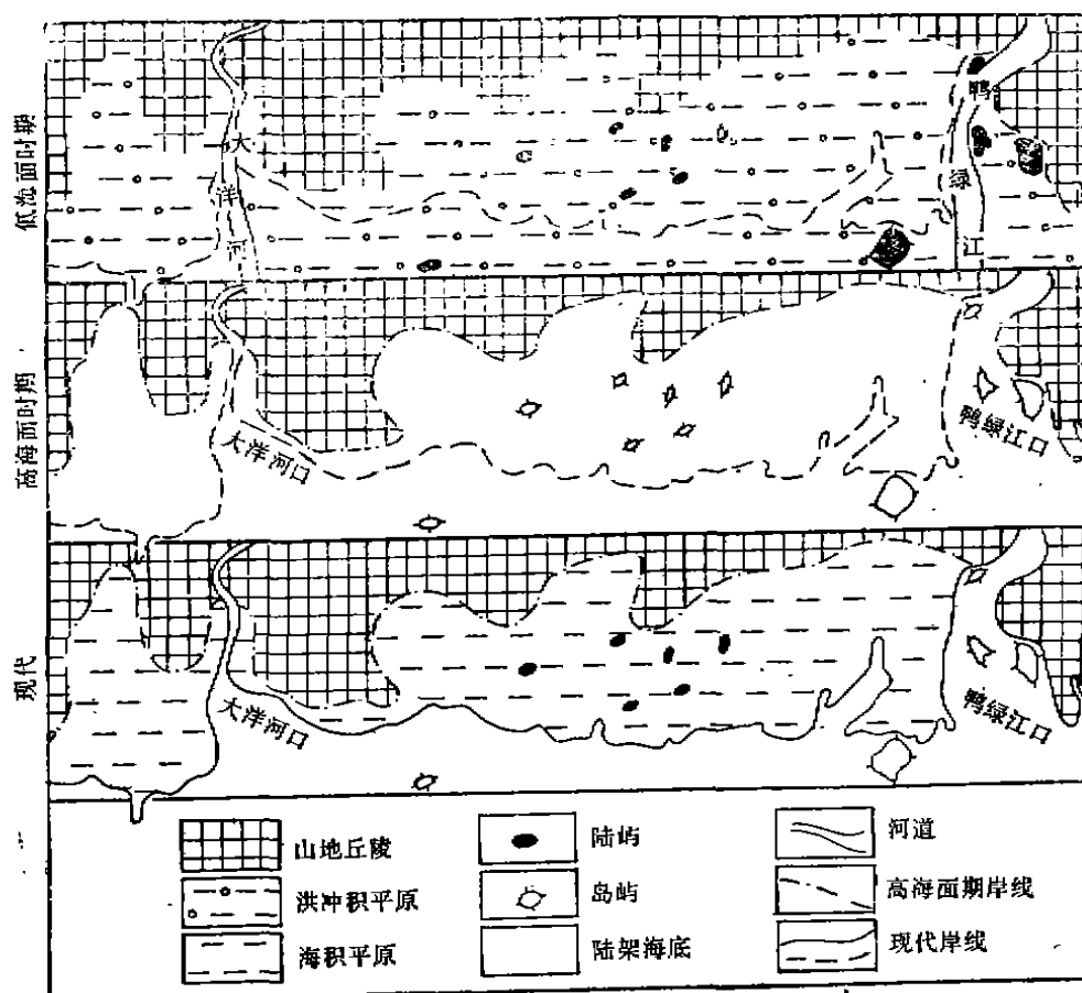
图 5 东沟平原晚冰期以来海岸环境演变
