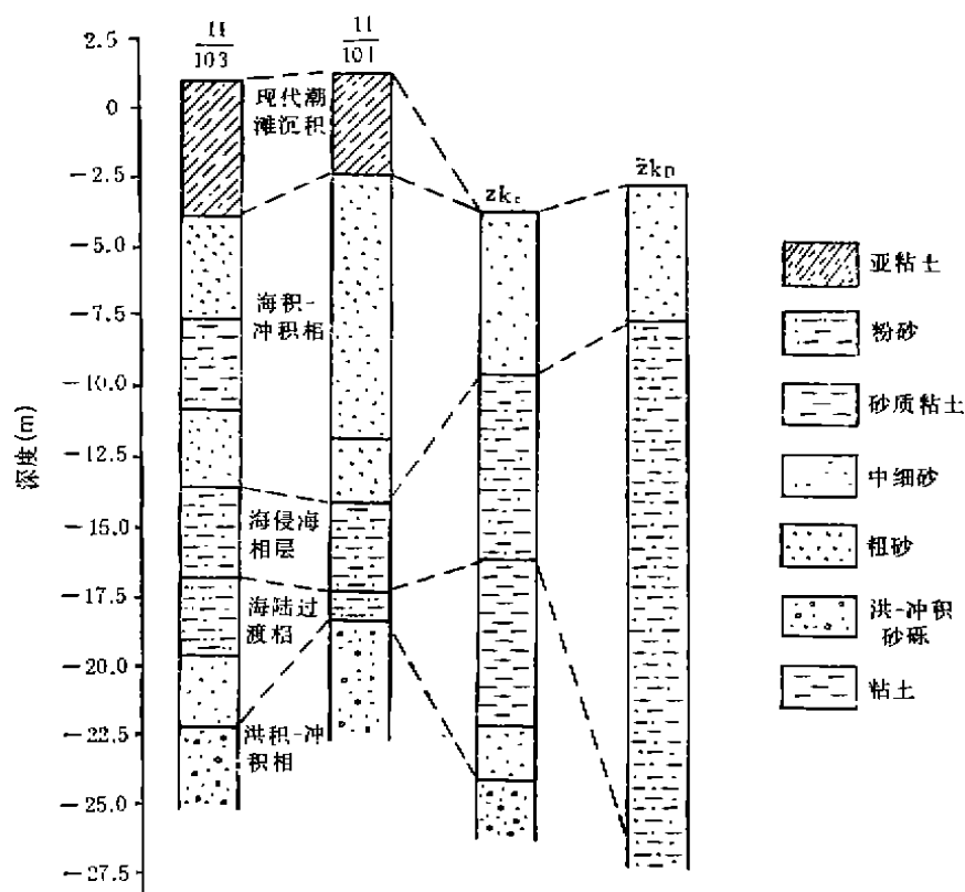
图 6 \frac{11}{103} , \frac{11}{101} 孔与 zk_C 、 zk_D 孔地层厚度对比图
