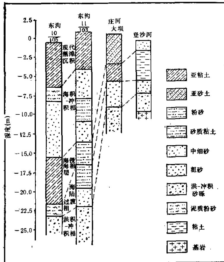
图2 辽东半岛东部海岸含洪积砂砾层的钻孔剖面图
