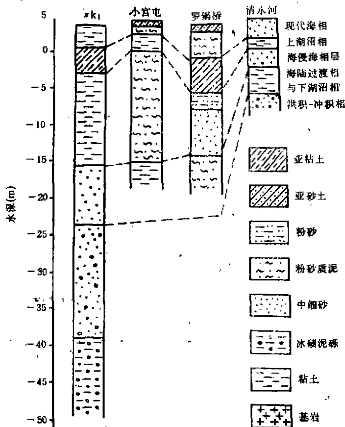
图3 辽东半岛东部含海相层的钻孔剖面
