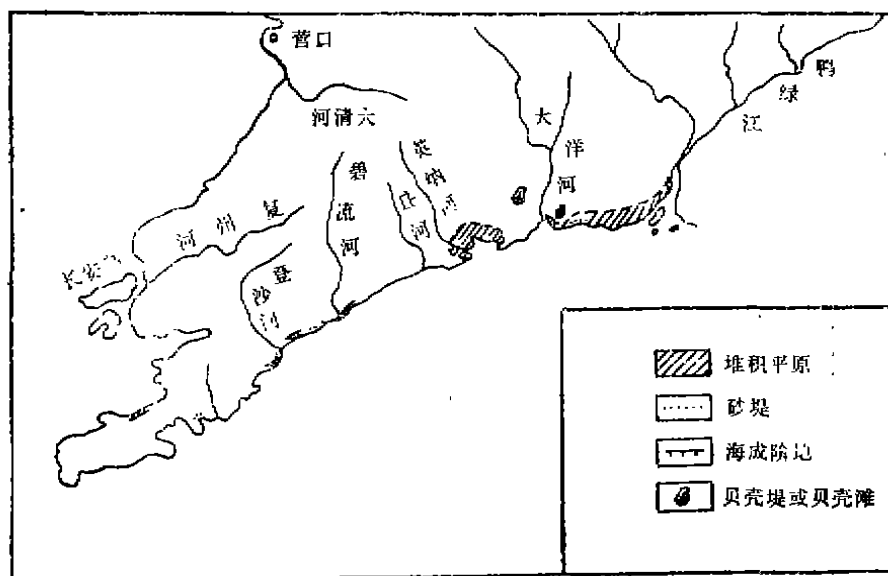
图1 辽东半岛东部海岸堆积地貌分布图
