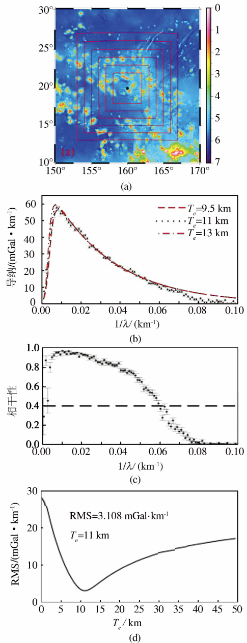
图 3 三维导纳分析算例
