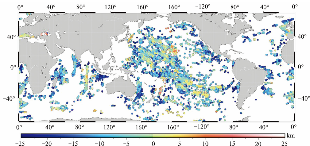
图8 本文计算结果与文献[10]结果之差
