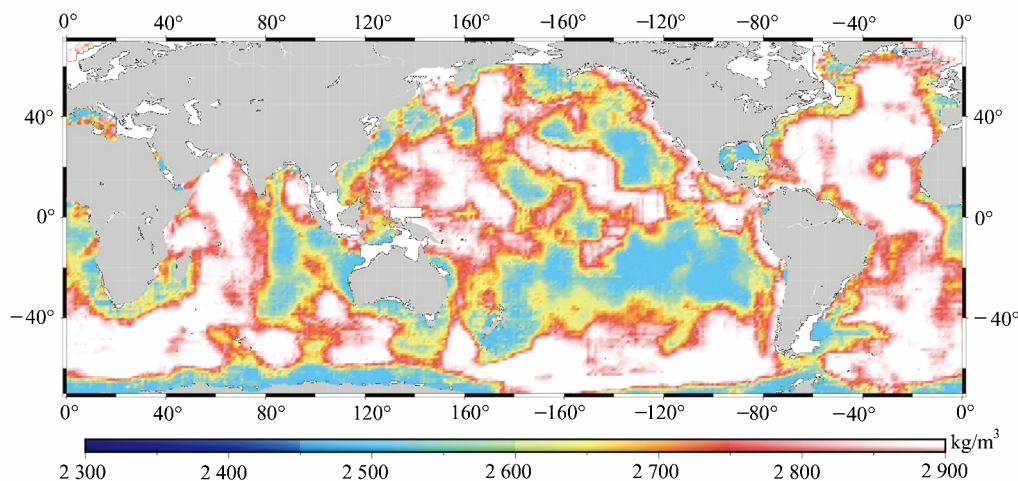
图 5 MWAT 方法计算海洋岩石圈有效弹性厚度时获得的洋壳密度参数
