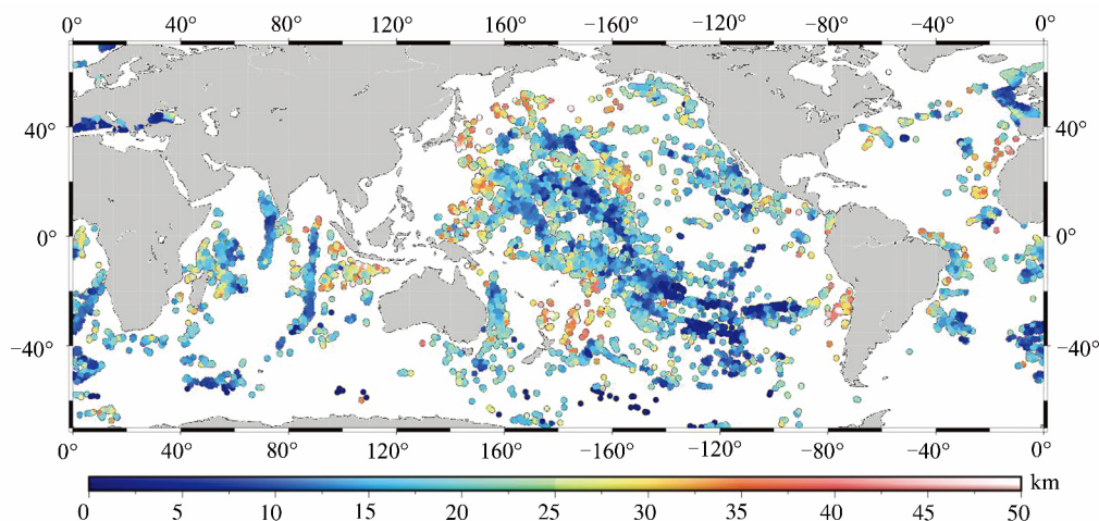
图7 全球海山底部岩石圈有效弹性厚度
