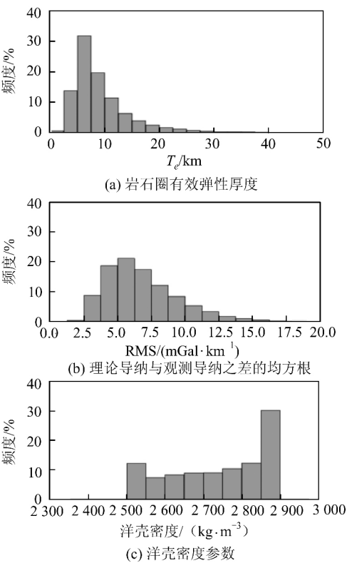
图 4 各参数的分布直方图 Fig. 4 Histogram of Parameters
