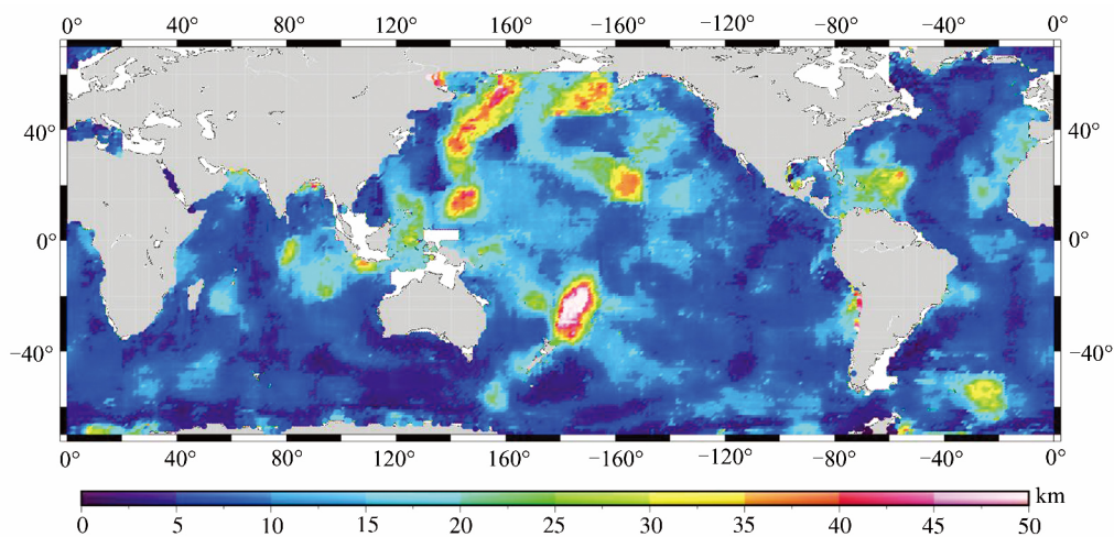
图 6 全球 1^{\circ} \times 1^{\circ} 海洋岩石圈有效弹性厚度模型
