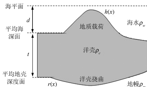
图1 海洋岩石圈挠曲均衡模型
