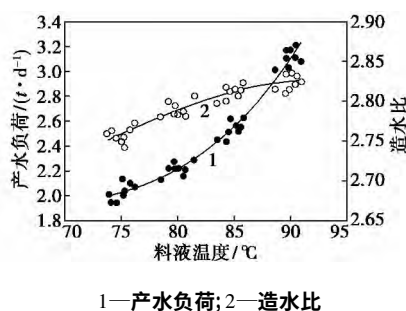
图7 料液温度对产水负荷与造水比的影响
