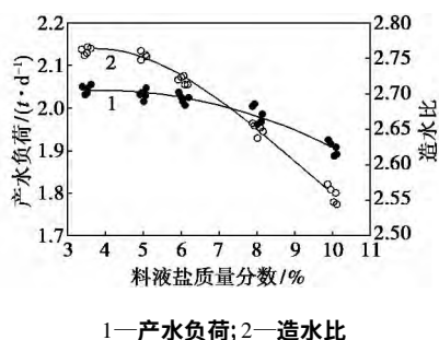
图 10 料液盐质量分数对产水负荷与造水比的影响
