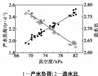
图8 渗透侧真空度对产水负荷与造水比的影响
