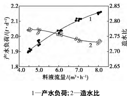
图9 料液流量对产水负荷与造水比的影响
