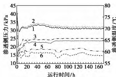
1—一效压力; 2—一效温度; 3—二效压力; 4—二效温度; 5—三效压力; 6—三效温度
